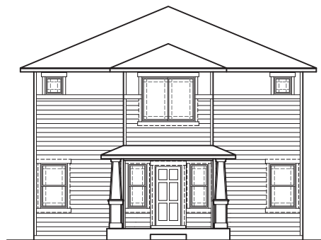
Elevation B
