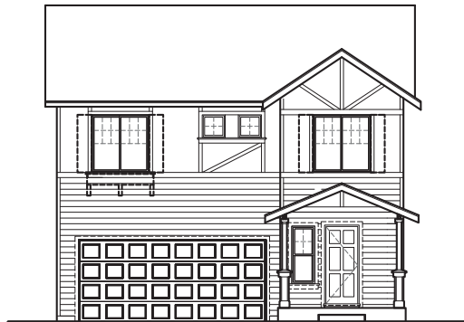
Elevation B
