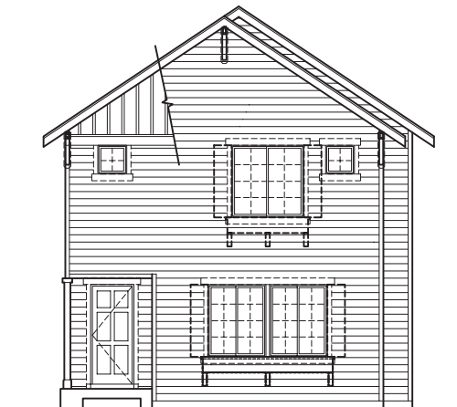
Elevation A
