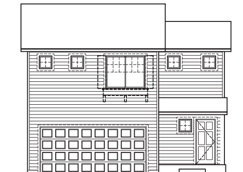
Elevation B
