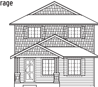
Elevation B
