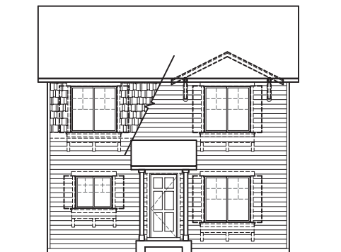
Elevation A
